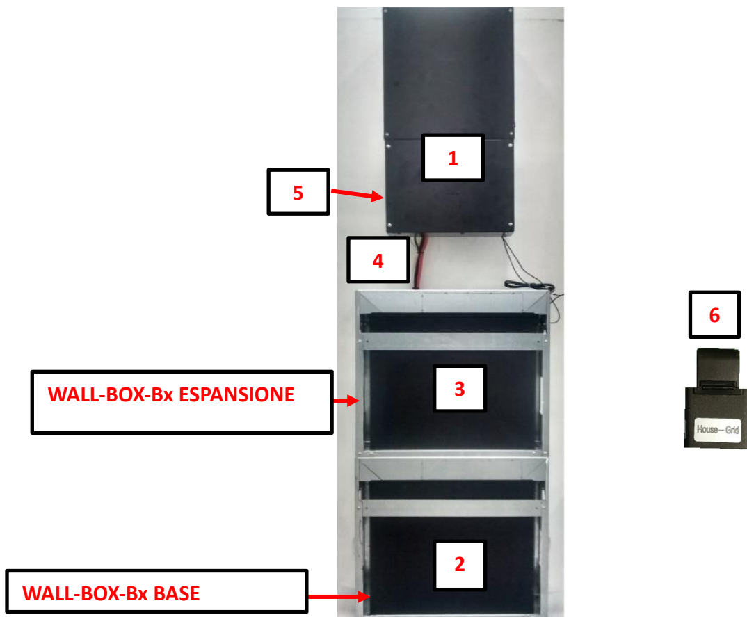
Figura 2 - Sistema M.STORE
