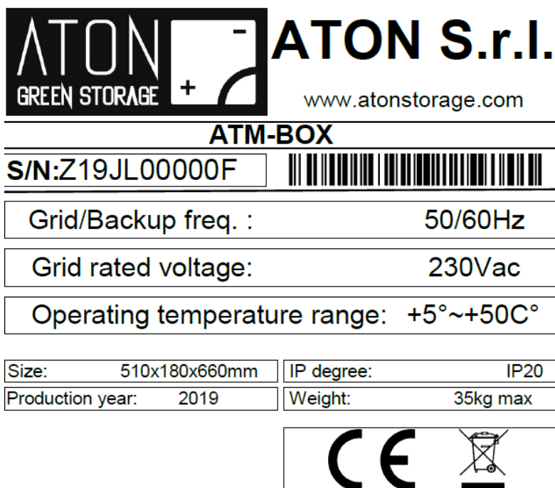
Figura 4 - Targa M.STORE
